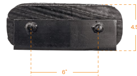
PROYECCIÓN Vista lateral solera.
